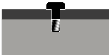
Fijación visible con tornillos en soportes de madera
